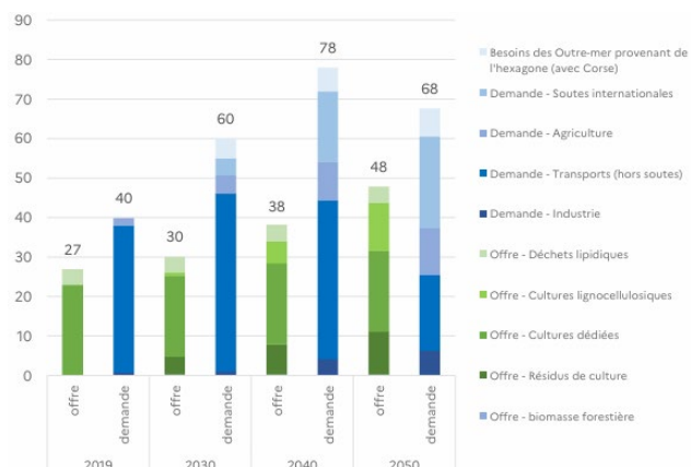
Fig. 9 - Demande (consommation primaire) et offre (production primaire) de biocarburants dans les modélisations du scénario de référence de la SNBC 3 (Sources : Bilan énergétique de la France, SDES, édition 2026 ; modélisations DGEC ; Périmètre France hexagonale et Corse ; TWh PCI)
