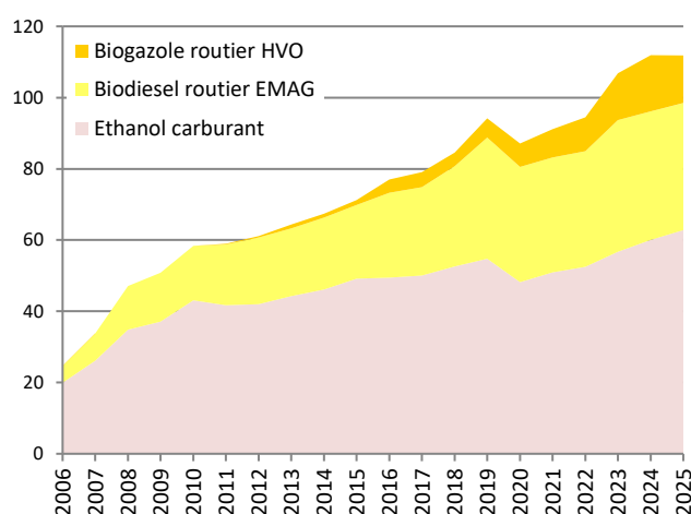
Fig. 3 - Evolution de la consommation mondiale de biocarburants dans les transports routiers en Mtep Source : IFPEN, d'après S&P Global
