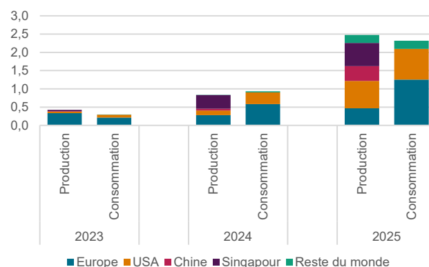
Fig. 6 -Evolution de la production et de la consommation de CAD par zone géographique (en Mtep).
