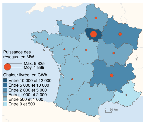
Figure 3.5.1.1 : puissance thermique et chaleur livrée par les réseaux de chaleur en 2019
