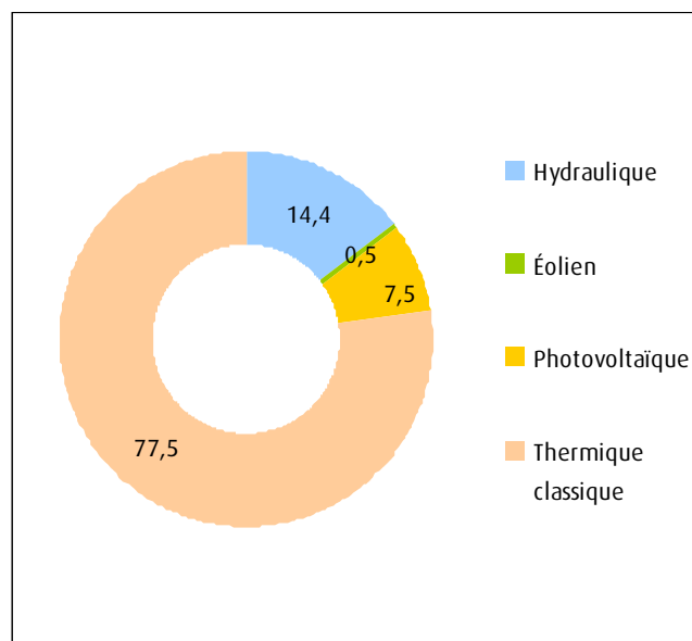
Figure 7.1.12 : structure de la production totale brute d'électricité à La Réunion (2 981 GWh en 2014)
