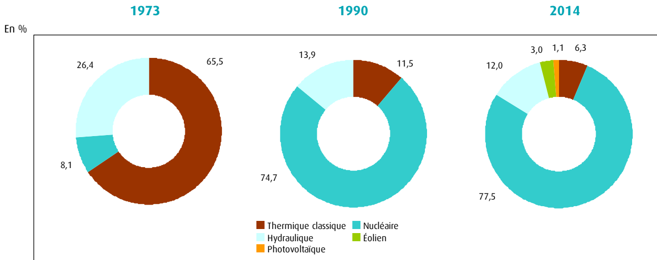
Figure 3.6.1 : structure de la production totale brute d'électricité
