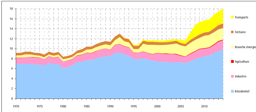
Figure 5.5.1 : consommation primaire d'énergies renouvelables thermiques et déchets par secteur
